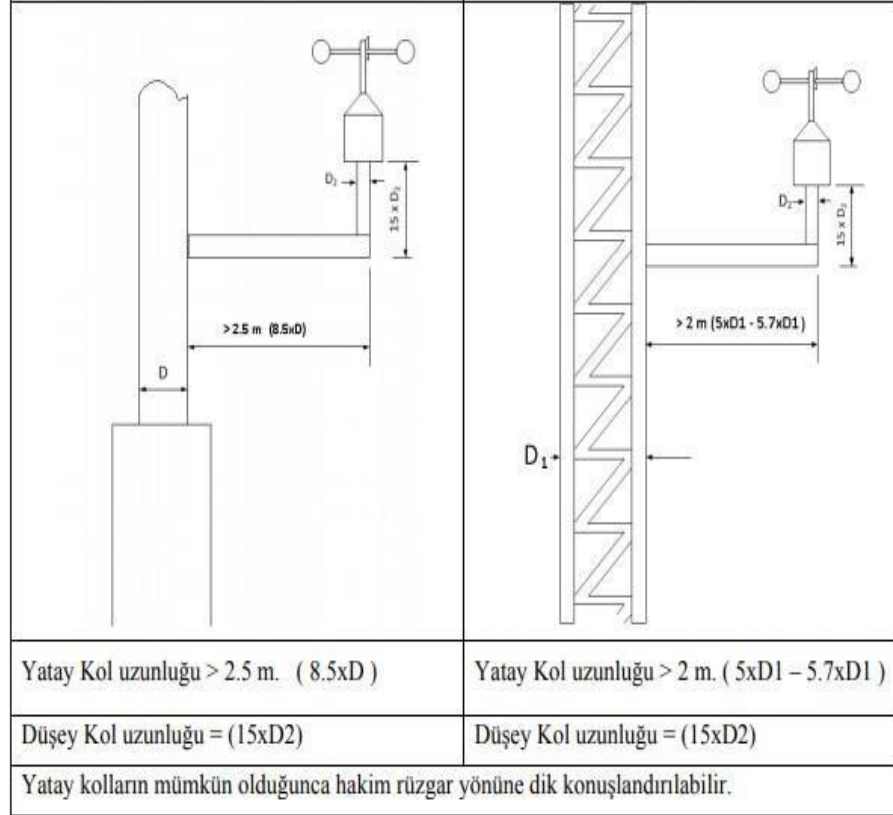
Şekil 2.18 Boru ve Kafes Tip Direk Standartları
