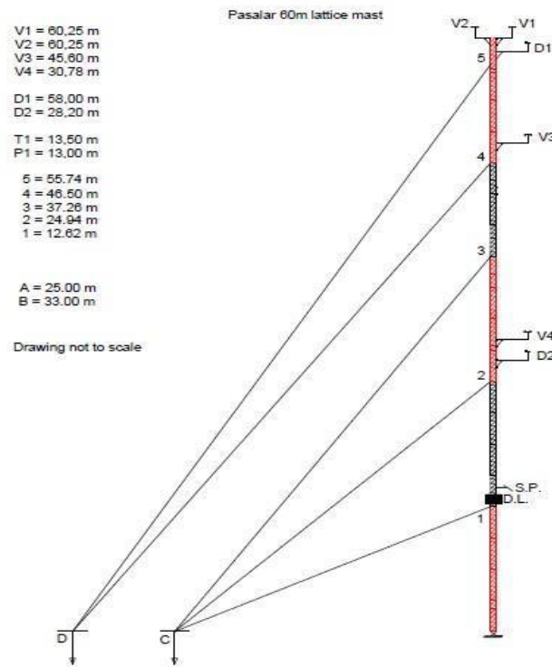
Şekil 2.22 60 Metrelik Ölçüm Direği Örnek Dizayını
