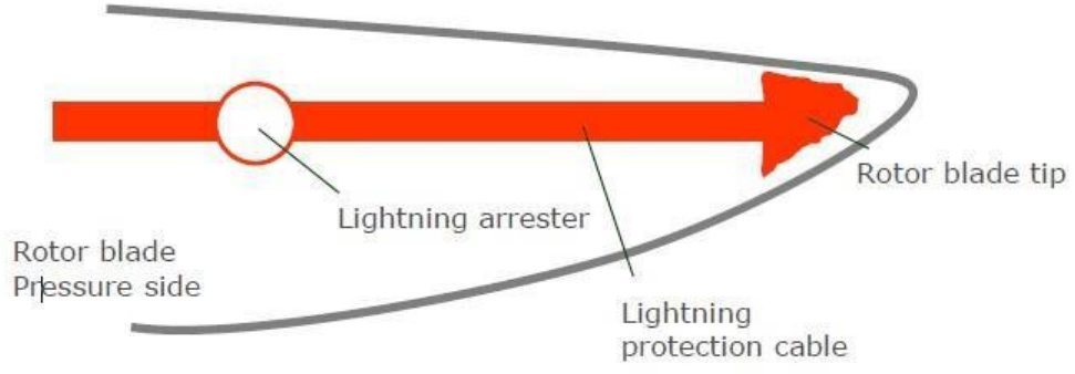
Şekil 5.29 Kanat Reseptörü
