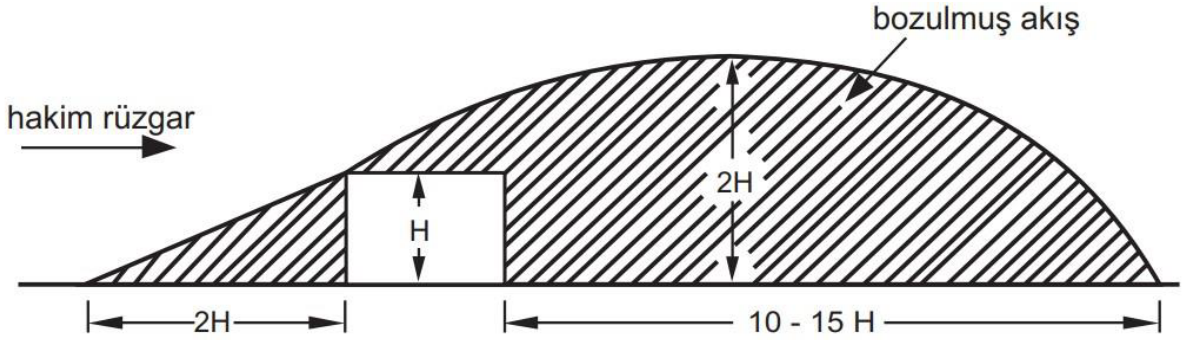
Şekil 1.19 Engel Etrafındaki Hava Akışı
