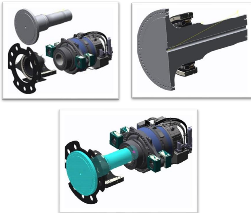
Şekil 5.17 Rotor Şaftı Görünümleri
