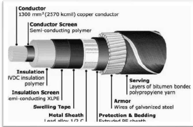
Şekil 13.12 Kablo
