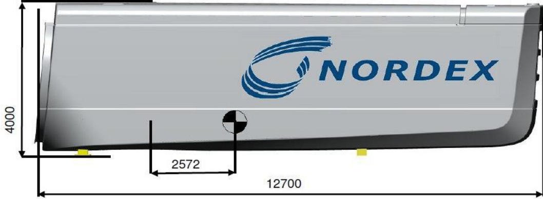
Şekil 5.6 Nacelle Boyutları
