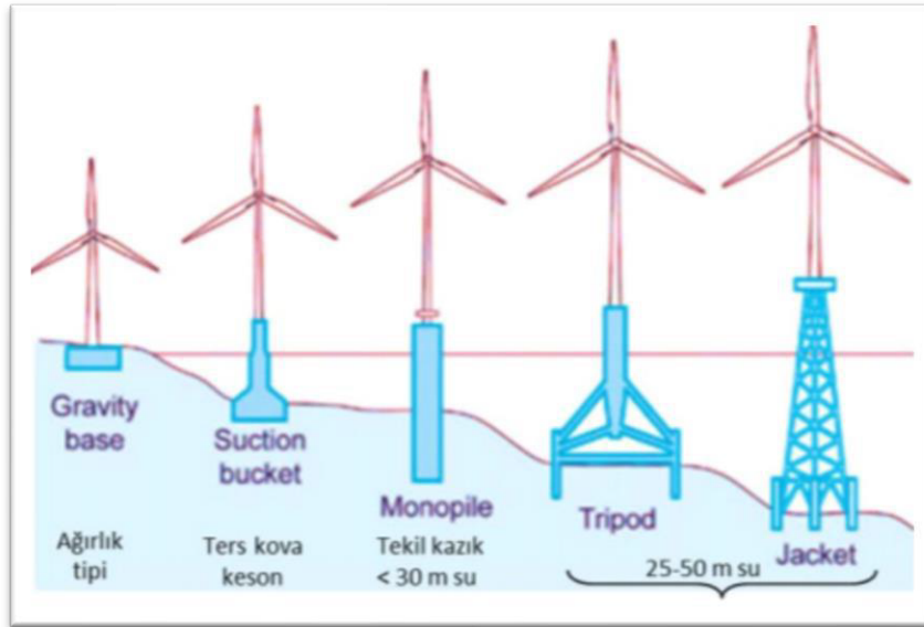
Şekil 13.4 Kule Tipleri
