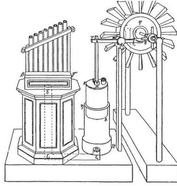
Şekil 4.1 Heron'un İlk Rüzgârla Çalışan Aleti (Org)
