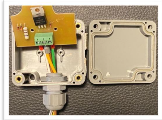
Şekil 2.10 Basınç Sensörü Dış ve İç Görüntüsü
