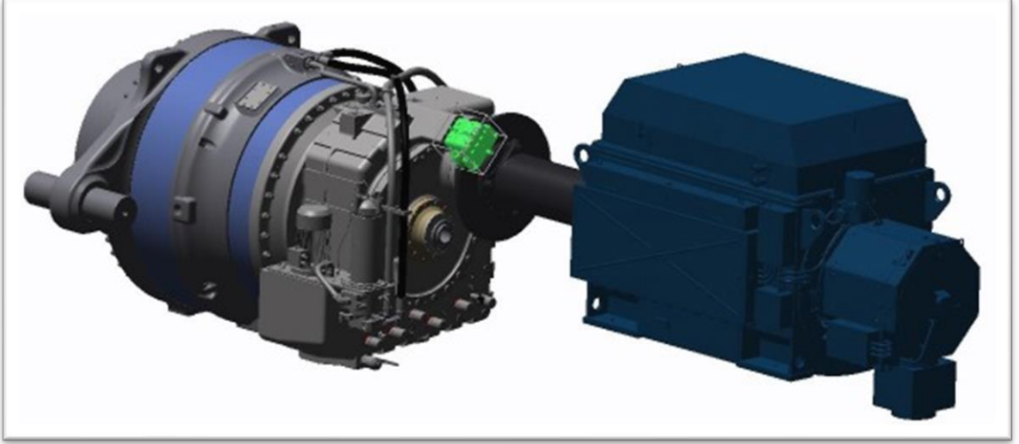
Şekil 5.20 Fren Sistemi
