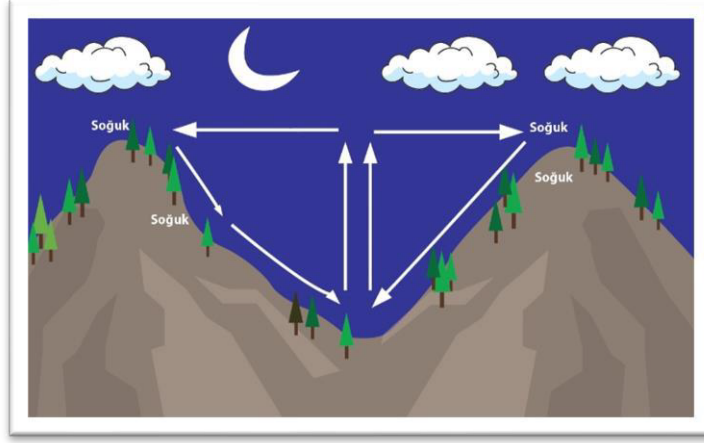
Şekil 1.11 Dağ Meltemi
