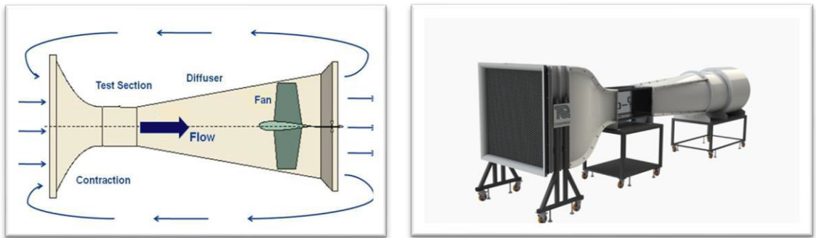
Şekil 2.15 Rüzgâr Tüneli
