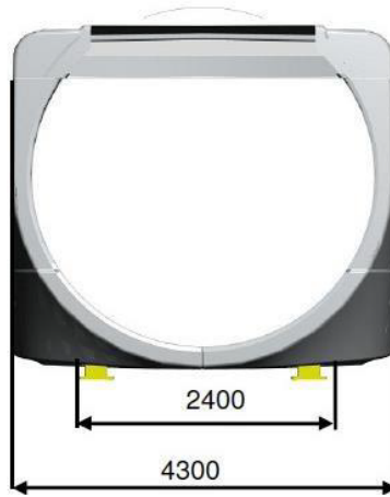
Şekil 5.7 Nacelle Ön Görünüş
