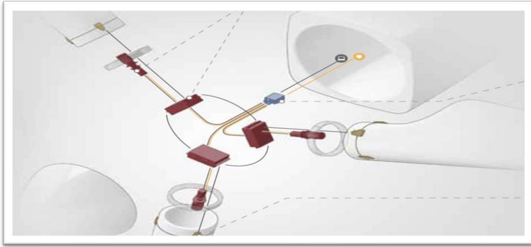
Şekil 5.25 Pitch Control
