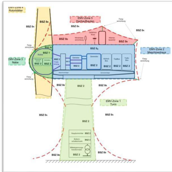
Şekil 5.28 Paratoner Sistemi
