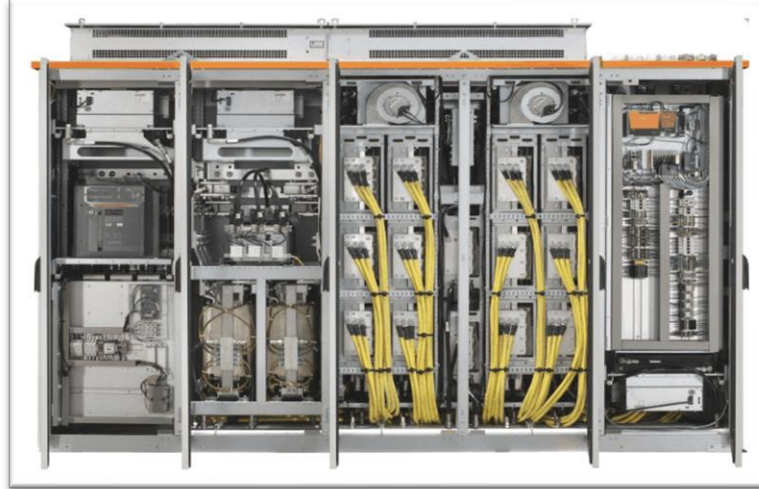
Şekil 5.16 Konvertör
