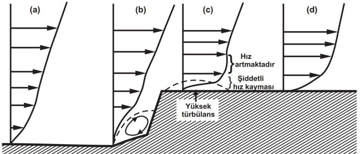
Şekil 1.26 Engeli Aşarken Rüzgâr Profiliinin Değişimi
