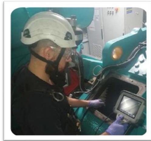
Şekil 7.2 Endoskopi İşlemi
