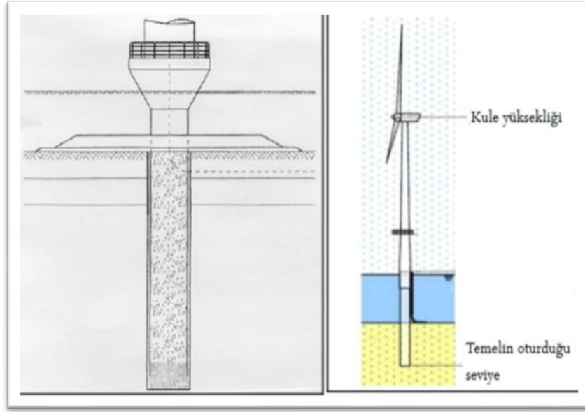
Şekil 13.5 Monopil Temel
