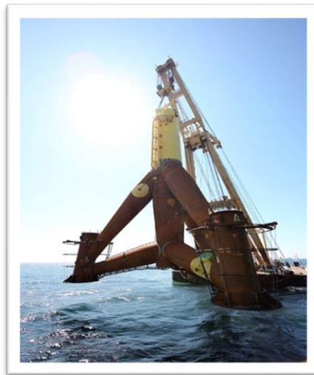
Şekil 13.8 Tripod Temel
