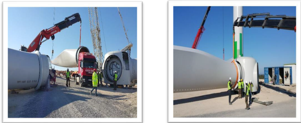
Şekil 6.40 HUB ve Yıldız Montajı
