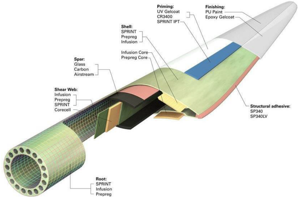
Şekil 5.23 Kanat Yapısı
