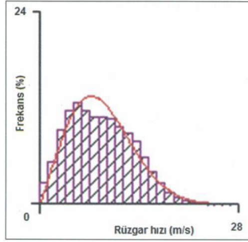
Şekil 3.17 Weibull Dağılımı
