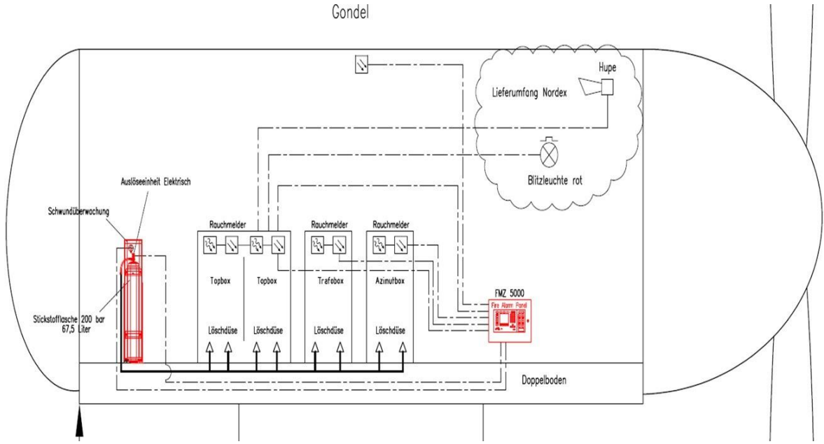
Şekil 5.42 Yangın Söndürme Sistemleri
