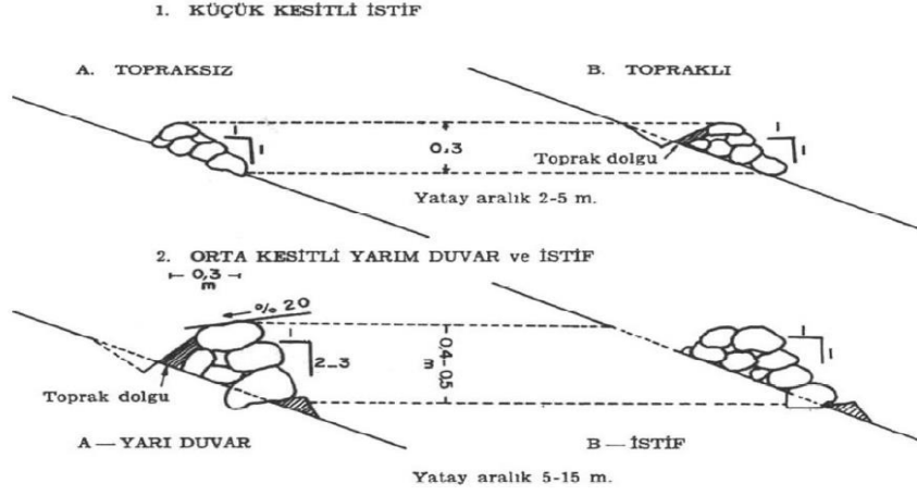
Şekil 10.14 Malzeme İstifleme Teknikleri
