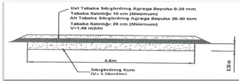
Şekil 6.4 Ulaşım Yolu Yapımı
