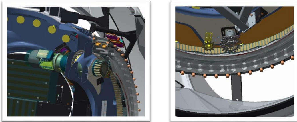
Şekil 5.26 Pitch Motorları
