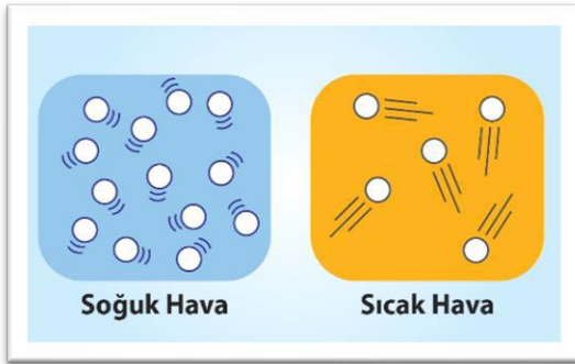
Şekil 1.3 Soğuk ve Sıcak Hava Hareketleri
