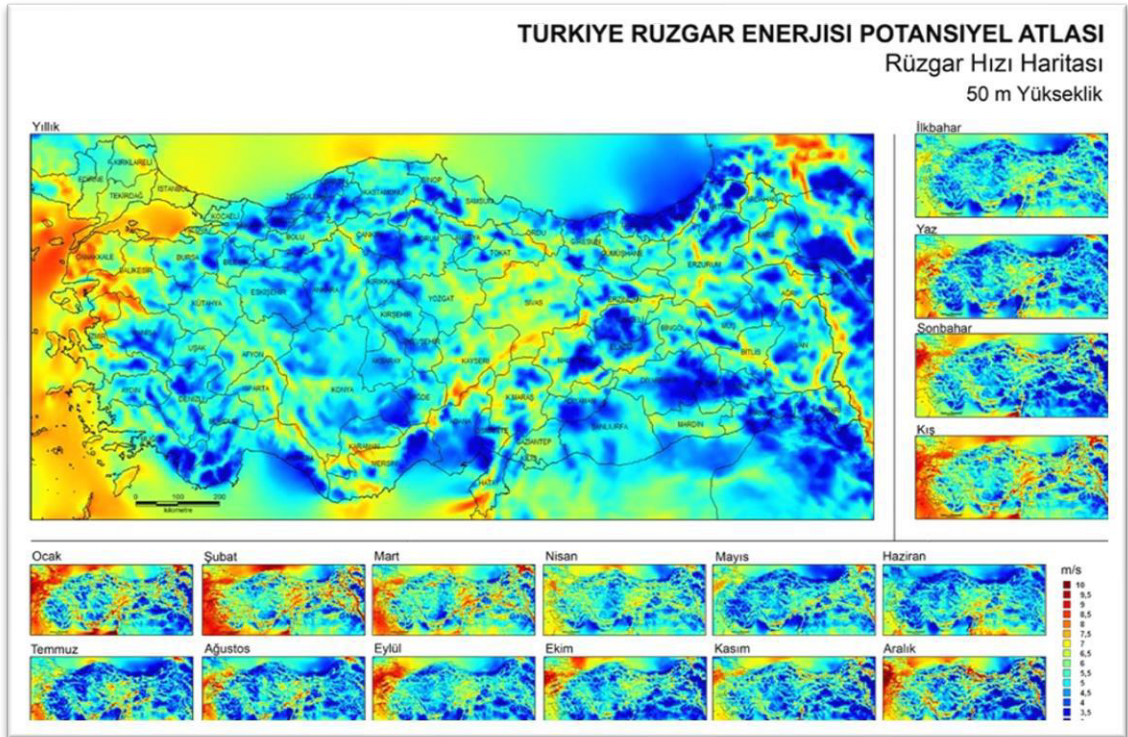
Şekil 3.5 Türkiye Rüzgâr Atlası
