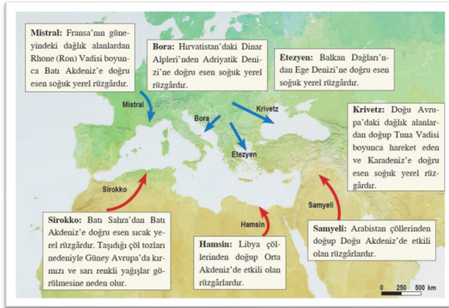
Şekil 1.13 Akdeniz Havzası'nda Esen Yerel Rüzgârlar
