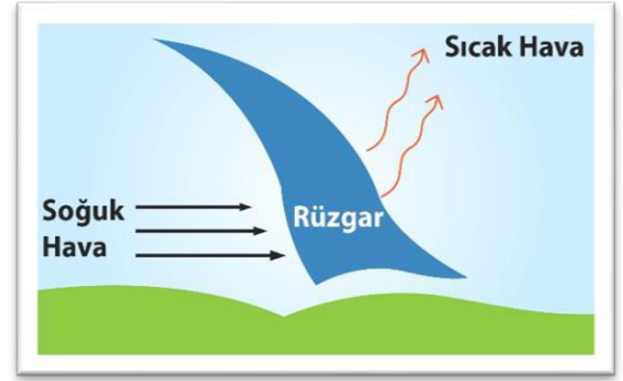
Şekil 1.2 Rüzgâr Oluşumu
