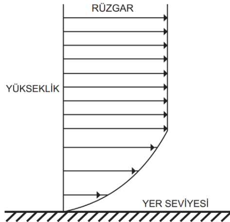
Şekil 1.17 Nötr Bir Atmosferde Rüzgâr Profili
