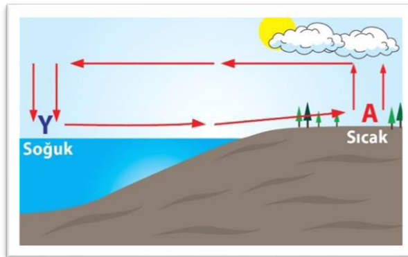
Şekil 1.8 Deniz Meltemi
