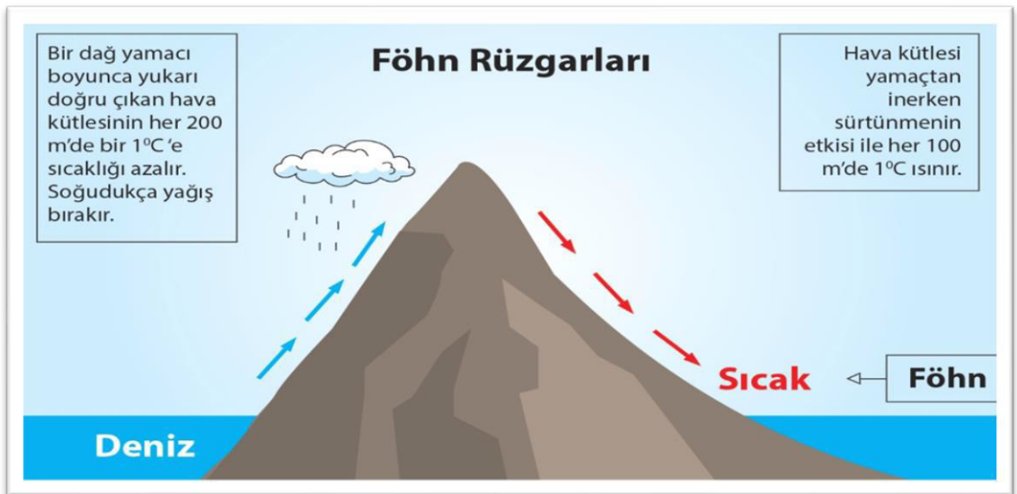
Şekil 1.12 Föhn Rüzgârları
